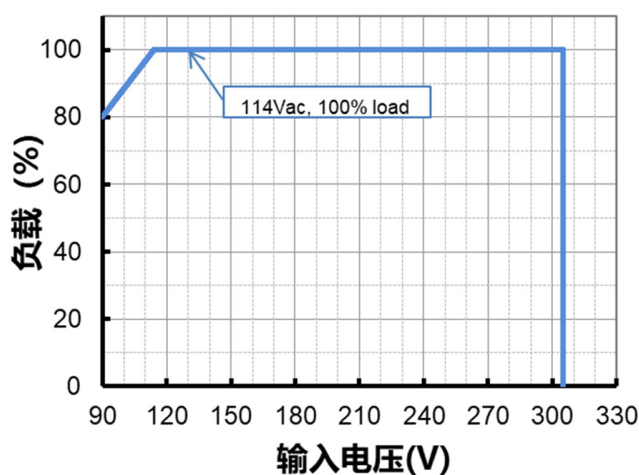
降额曲线
