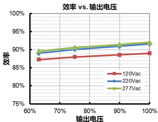
EUW-150D320Dx (Io=2800mA)
