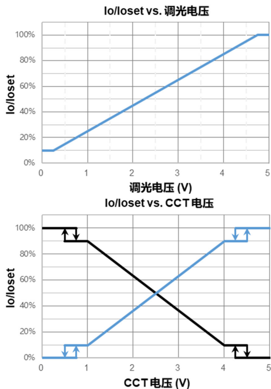
示意图 1：正逻辑
