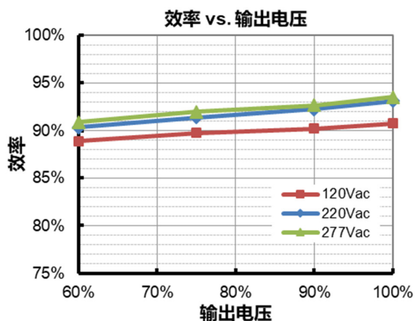
EUW-150D140Dx (Io=1050mA)
