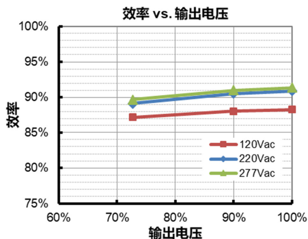
EUW-150D320Dx (Io=3200mA)
