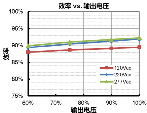
EUW-150D140Dx (Io=1400mA)
