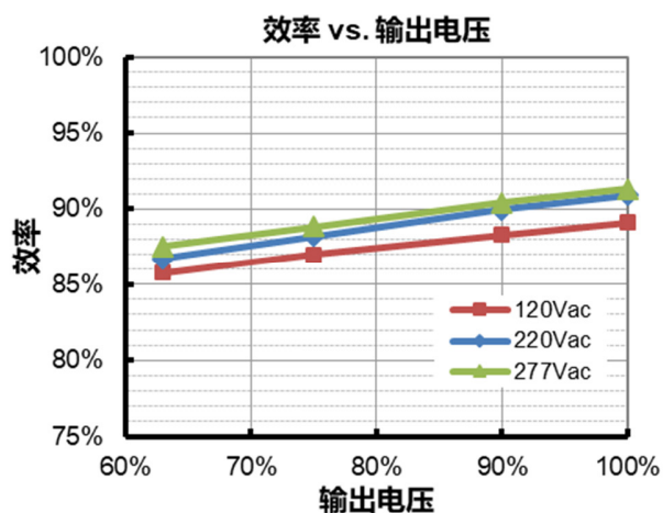
EUW-100D210Dx( I_o=1850\text{mA} )
