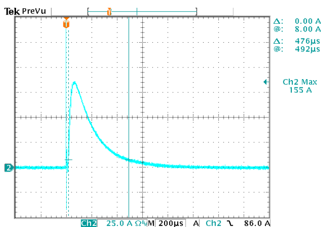
EUW-100D105Dx( I_o=700\text{mA} )
