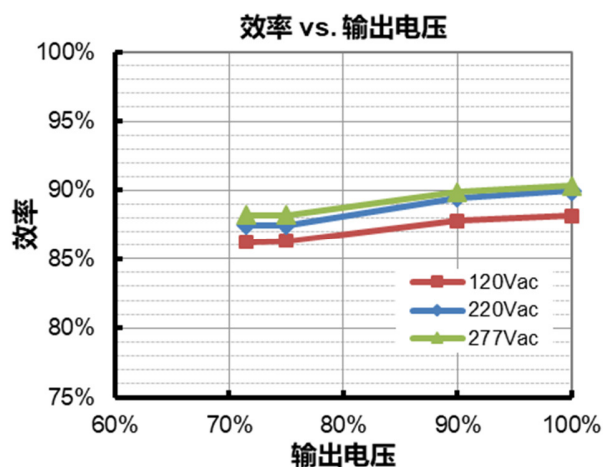
EUW-100D210Dx( I_o=2100\text{mA} )
