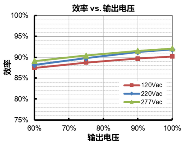
EUW-100D105Dx( I_o=700\text{mA} )
