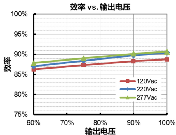
EUW-100D105Dx( I_o=1050\text{mA} )
