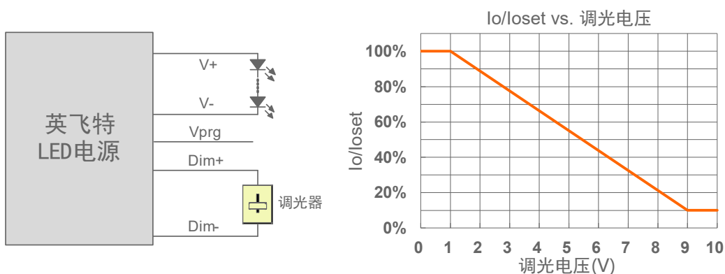
示意图 4：负逻辑
