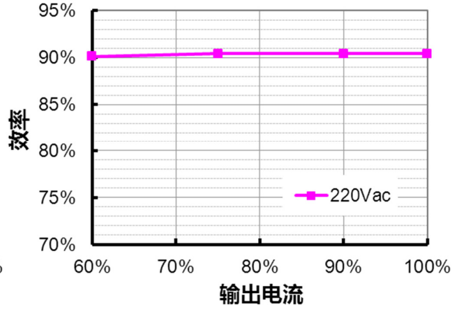
EBV-060S048SV 效率 vs. 输出电流
