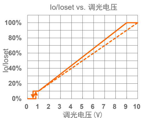
示意图 1：正逻辑
