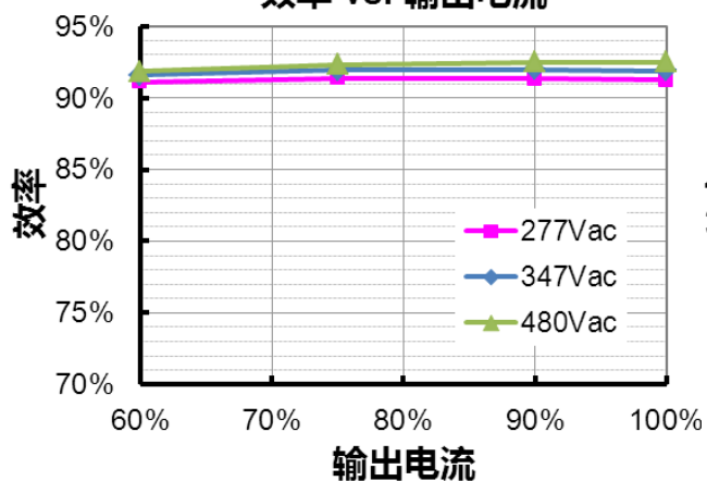
ESV-320S048SV 效率 vs. 输出电流
