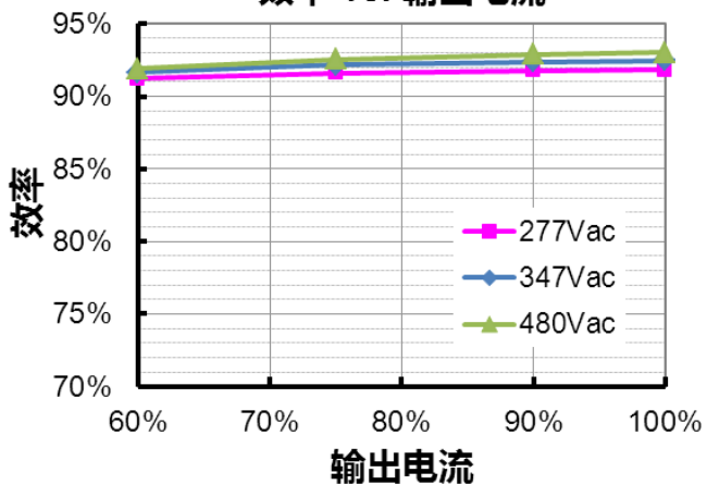
ESV-320S048SV 效率 vs. 输出电流
