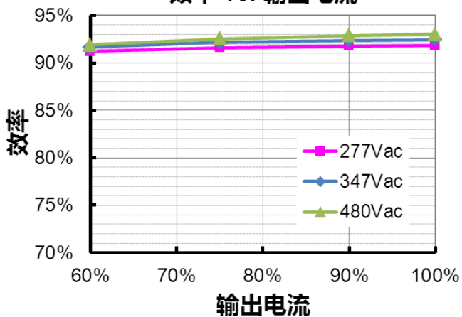
ESV-320S048ST 效率 vs. 输出电流
