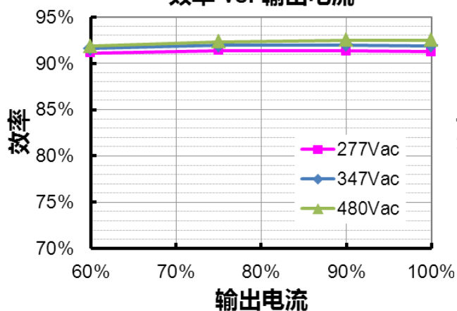
ESV-320S048ST 效率 vs. 输出电流
